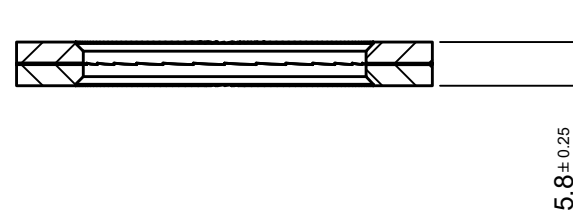
A-A (1 : 1)
